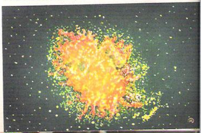
FIG. 18. LA NEBULOSA DEL CANGREJO que aparece en la constelación de Taurus, está constituida por los restos de una estrella que hizo explosión (supernova) hacia el año 1054 antes de Cristo. La explosión fue observada entonces por los astrónomos chinos. (Dibujo basado en una fotografía del Observatorio de Monte Palomar.)
