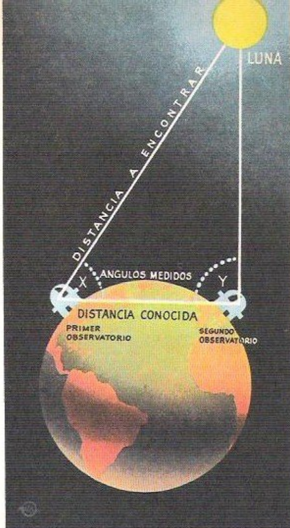
FIG. 38. COMO ES MEDIDA LA DISTANCIA ENTRE LA TIERRA Y LA LUNA. La distancia entre la tierra y la luna puede ser medida por dos astrónomos situados en distintos lugares de nuestro planeta. Los datos que necesitan determinar son los ángulos en los cuales ven la luna en el mismo momento desde sus observatorios respectivos y la distancia que separa ambos observatorios. En ese caso tienen un lado y dos de los ángulos de un triángulo; con estos datos se puede obtener, mediante una operación sencilla, la longitud de los otros dos lados, que representan la distancia entre la tierra y la luna, tal como se observa en el diagrama. Para medir la distancia entre la tierra y una estrella el procedimiento es semejante, sólo que por las enormes distancias que separan las estrellas de la tierra, cuando una estrella es observada en el mismo momento, desde dos puntos distintos, no presenta ángulos diferentes. Los astrónomos descubrieron, sin embargo, que si observan una estrella una noche y la observan seis meses después, los ángulos son diferentes. Como en esos seis meses la tierra ha cubierto la mitad de su recorrido anual en torno al sol y se encuentra a 297 500 000 Km del lugar donde se encontraba seis meses antes, disponen también de los tres datos necesarios para encontrar los lados del triángulo, o sea, la distancia de la estrella a la tierra. Con este método puede calcularse la distancia de cualquier estrella que esté a menos de 300 años-luz de la tierra.
