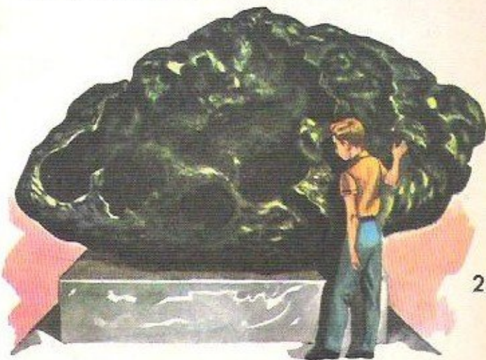
FIG. 30. EL METEORITO DE VILLAMETTE fue encontrado cerca de Oregón City, E.U., en 1902, y es conservado en el Museo de Historia Natural de New York. Pesa 15,5 toneladas. (De una fotografía).
