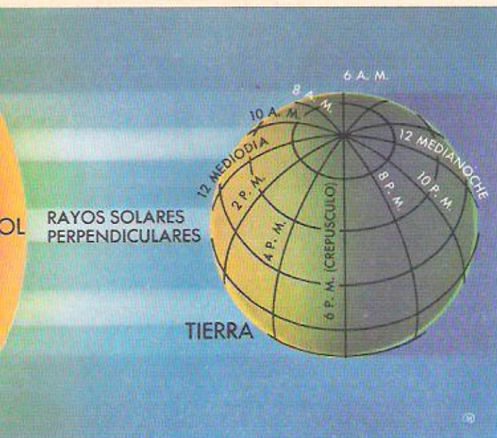
FIG. 95. LAS HORAS SE SUCEDEN debido al movimiento de rotación de la tierra.
