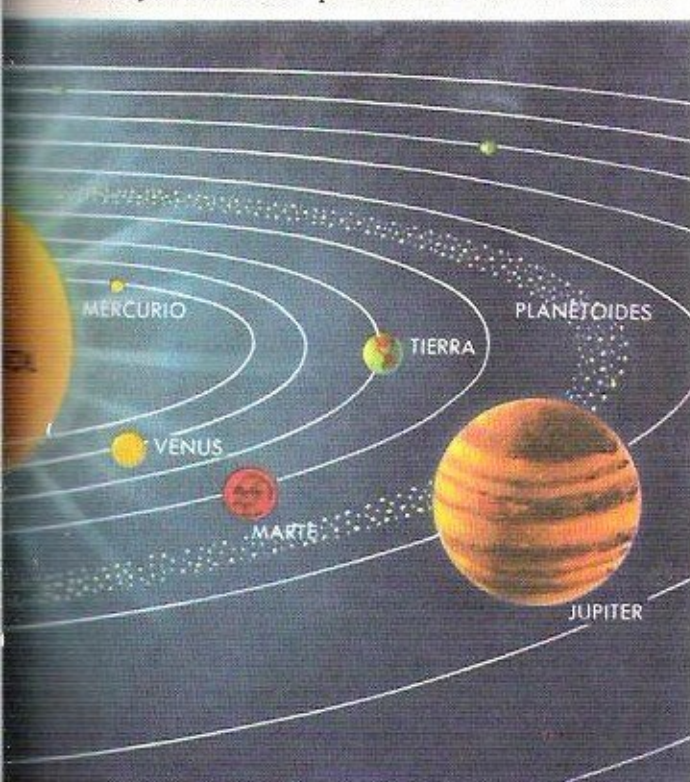
FIG. 25. LOS PLANETOIDES o asteroides se encuentran entre las órbitas de Júpiter y Marte, como puede verse en el diagrama. Han sido descubiertos en su mayor número por medio de fotografías y se conocen hasta ahora unos 1 500. Ninguno es visible sin el empleo del telescopio. Algunos de los planetoides penetran entre las órbitas de Marte y la Tierra, y uno de ellos, Eros, se encontrará a una distancia de unos 22,4 millones de Km de la tierra en el año 1975.
