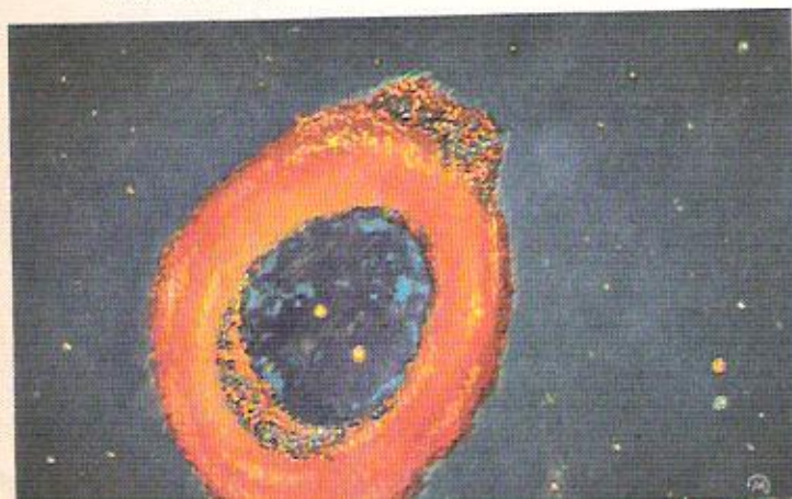
FIG. 17. LA NEBULOSA DE LIRA, del tipo denominado anular o planetaria, está formada por una envoltura gaseosa iluminada por la débil luz de una estrella central. Se cree que esta nebulosa se originó en una «explosión» estelar registrada hace millares de años. (Dibujo basado en una fotografía del Observatorio de Monte Palomar.)
